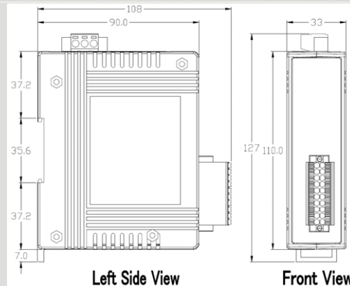
Dimensions
